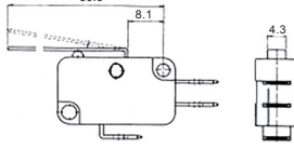
Long lever
